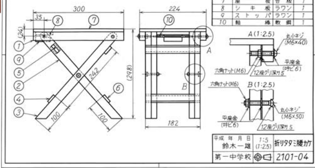
19回 折りたみ腰かけの組立図
