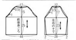
図17 スモックの型紙のつくり方の例 (3-4歳児 単位cm)
