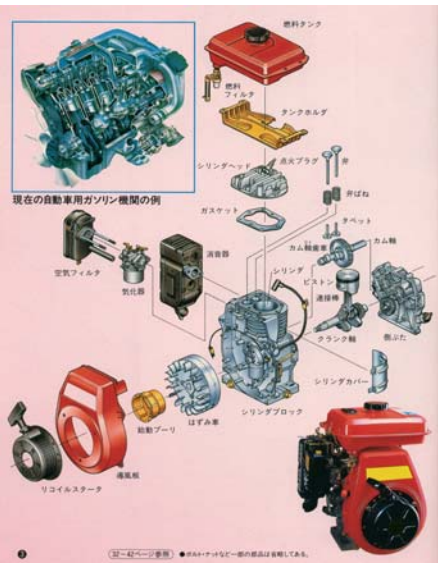
図16 現在の自動車用ガソリン機関の例
